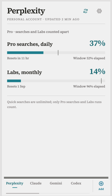
4e Perplexity
