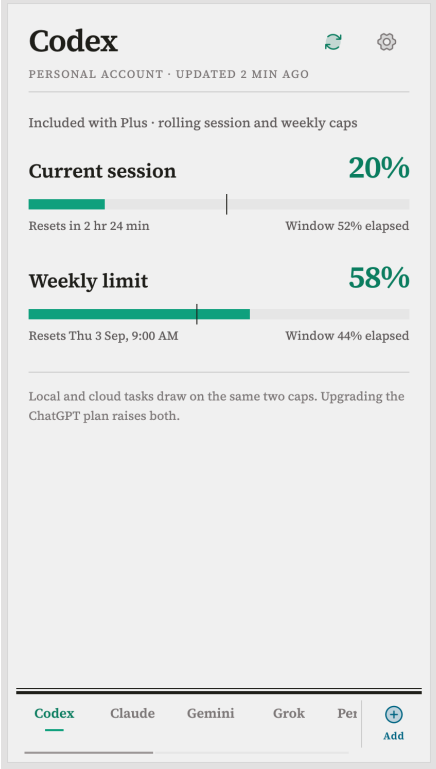
4c Codex
