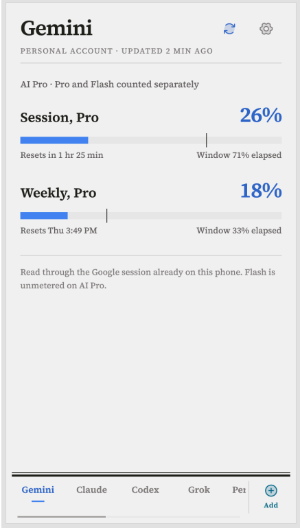
4b Gemini
