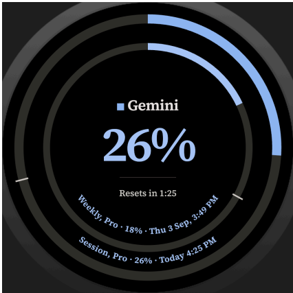
4b Gemini
