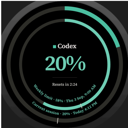
4c Codex
