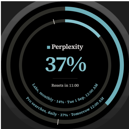
4e Perplexity
